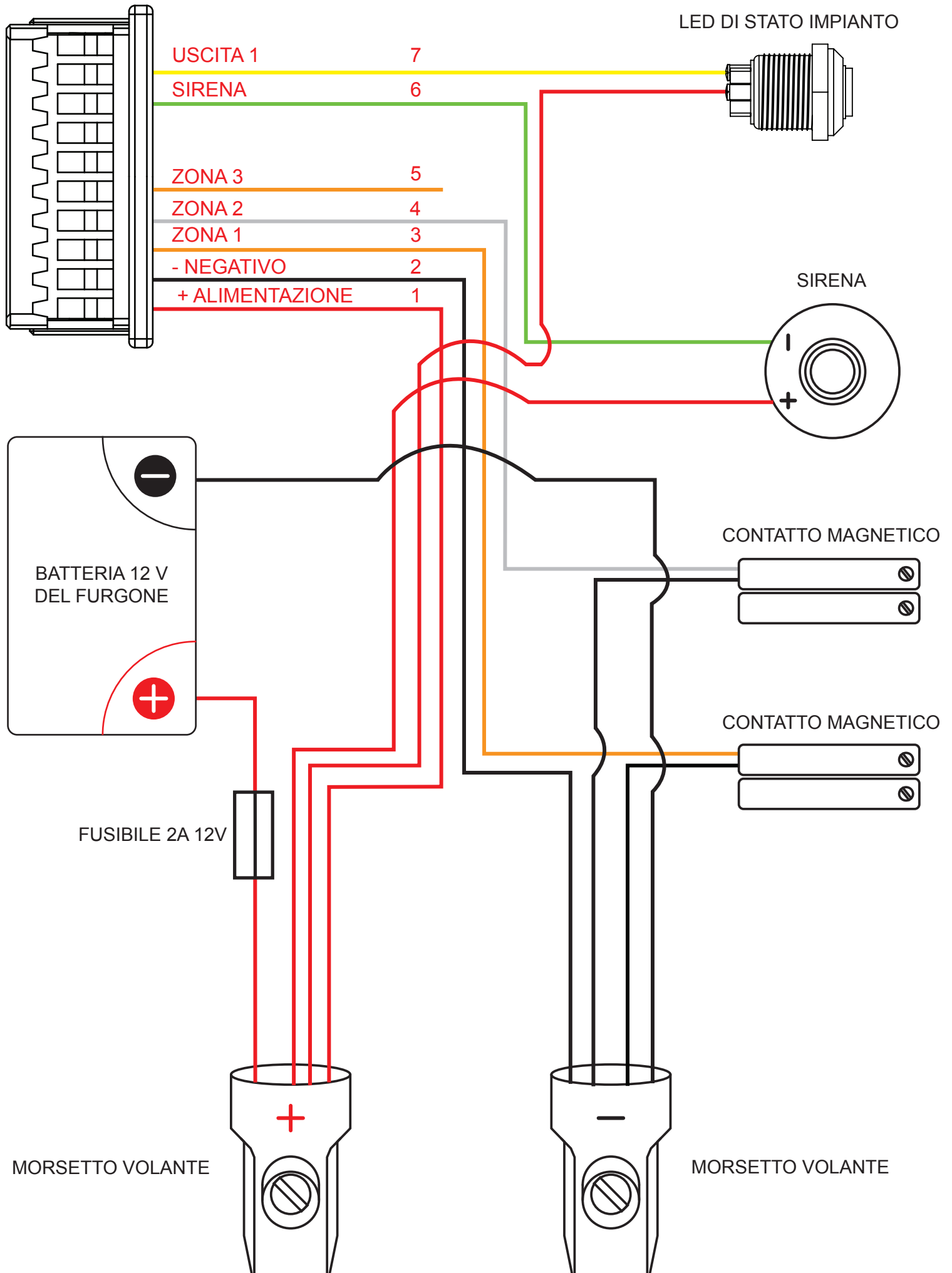
Schema di collegamento di FURGO-GSM
